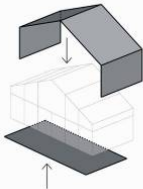
FACHADAS E-O Y CUBIERTA DE VIROC
